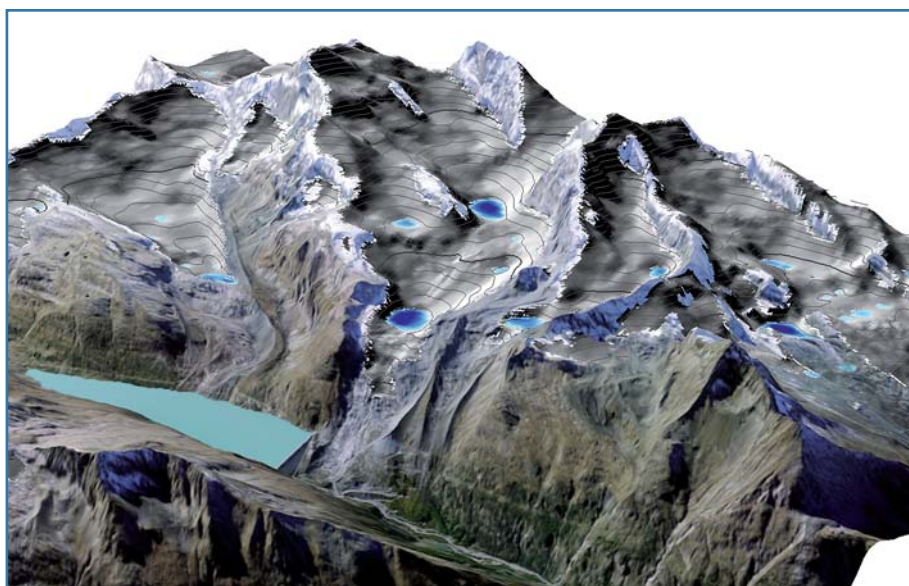
Bild 11. Die modellierten Gletscherbetten der Region Mattmark. In der Bildmitte das Bett des Allalingletschers mit zwei grösseren modellierten Überflutungen (potenzielle Seen). Reproduziert mit Bewilligung von swisstopo (BA110005).
