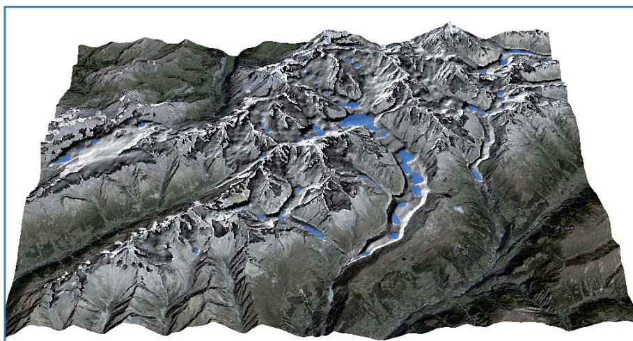
Bild 10. Überblick über die Region um den Aletschgletscher. Dargestellt sind die modellierten Gletscherbetten (die Gletscher vollständig entfernt) mit den darin detektierten Überflutungen (potenzielle zukünftige Seen). Reproduziert mit Bewilligung von swisstopo (BA110005).
